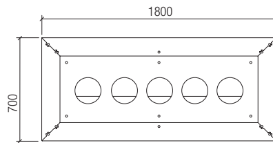
W 18/7 ng 1800 x 700 mm
